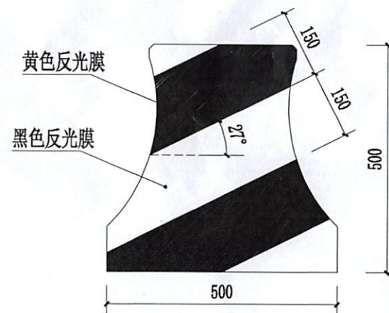
护栏端头反光立面标记图
