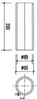
伸缩缝处栏杆接头构造
