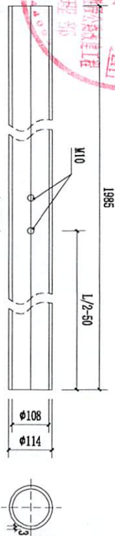
栅栏构造图
