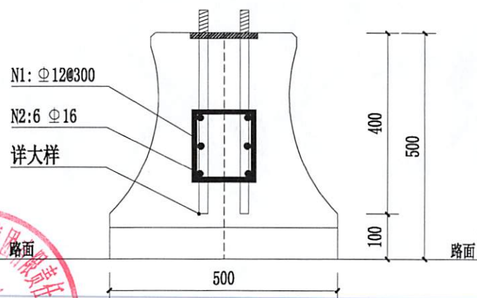
防撞护栏钢筋结构图
