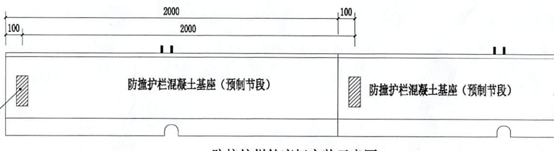
防撞护栏轮廓标安装示意图
