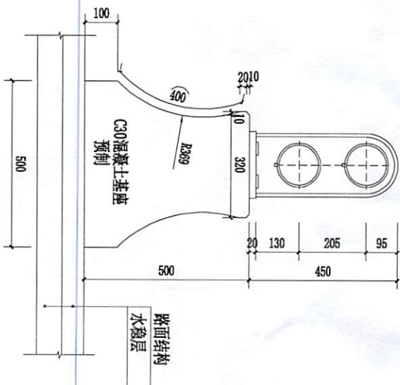
隔离墩构造图
